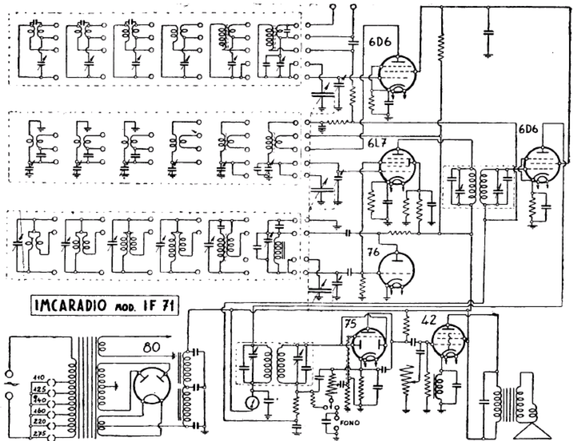
— IMCARADIO. — Mod. « IF 71 ». — Produzione 1937. — Media frequenza: 467 kHz.
